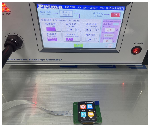
图 5-2 ESD 测试图
