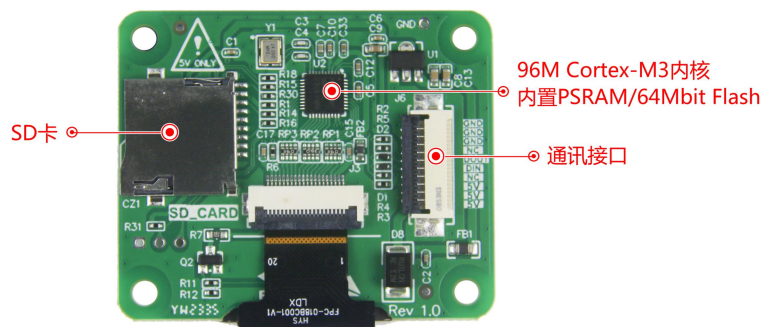
图 1-2 硬件配置图
