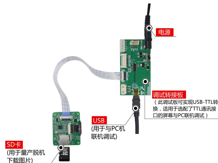
图 1-3 调试工具图
